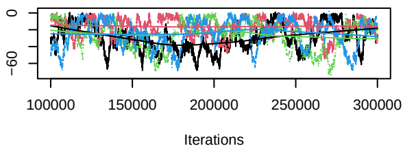
Trace of d.III.chemo_antiangio
